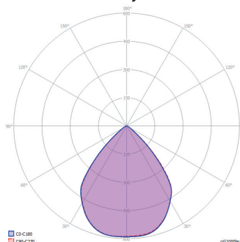
90° fényterelő
